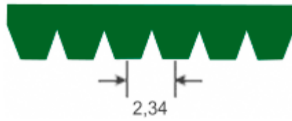
Correia passo 2,34 mm X 3,30 mm
